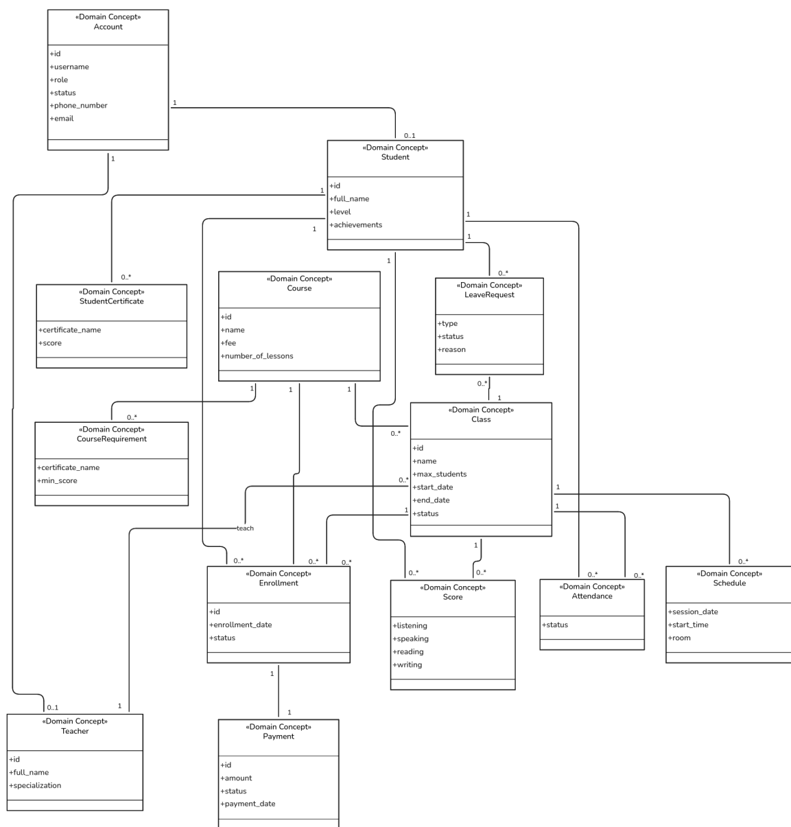
Hình 68: Biểu đồ Mô hình miền
